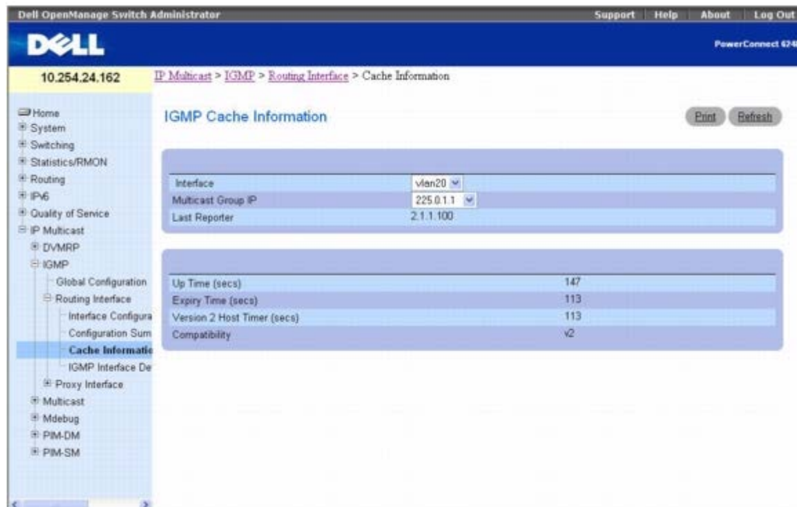
图 13-10. IGMP 高速缓存信息
